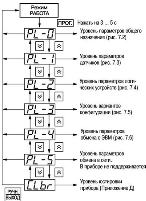
Рисунок 6.1 – Схемы выбора уровня программируемых параметров
