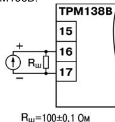
Рисунок 3.4 – Схема подключения датчика с токовым входом
