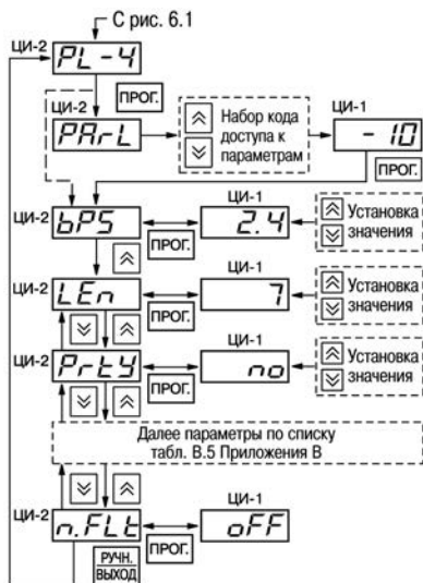
Рисунок 7.6 – Схема установки программируемых параметров на уровне PL-4
