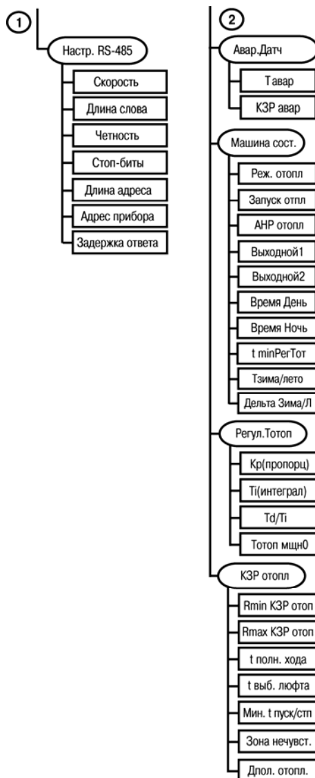
Рисунок И.1 – Главное меню прибора (продолжение)
