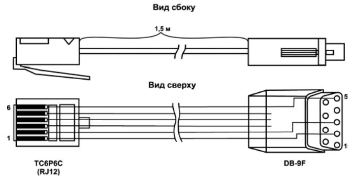
Рисунок Д.2 – Схема кабеля KC2
