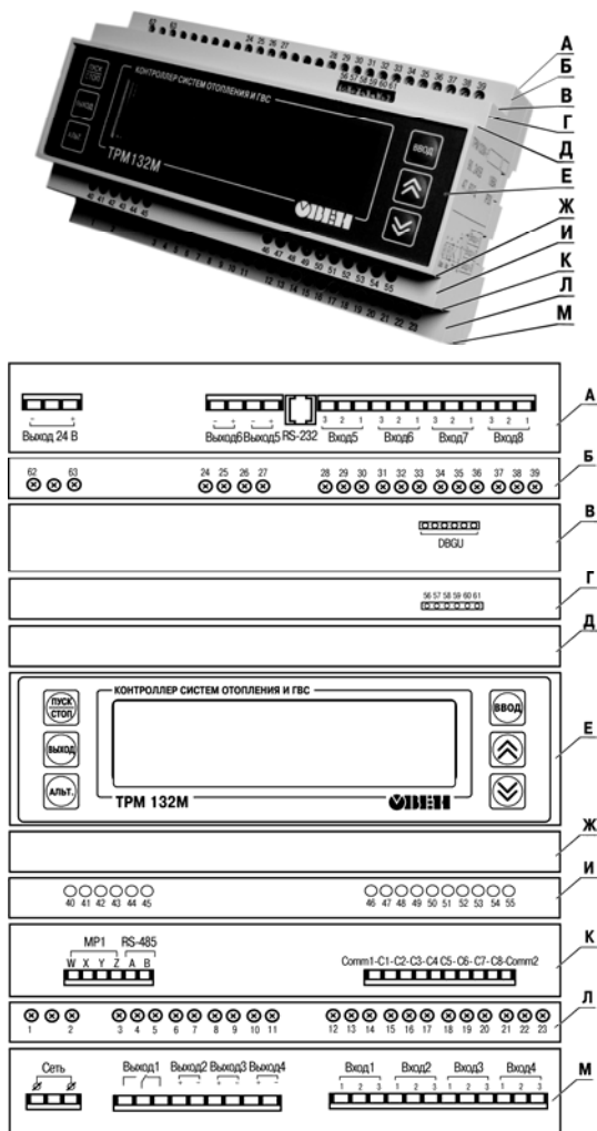
Рисунок 3.1 – Прибор TPM132M-01: внешние связи, элементы индикации и управления
