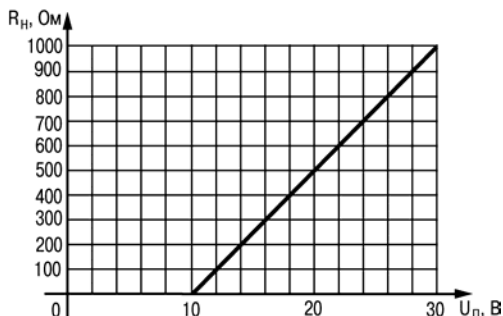
Рисунок 3.7 – График зависимости R_n ( U_n )
