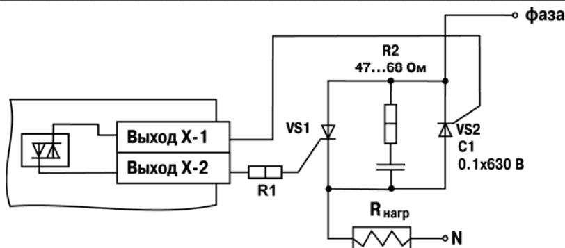
Рисунок Б.11 – Схема подключения нагрузки к ВУ типа С двух тириستоров, подключенных встречно-параллельно
