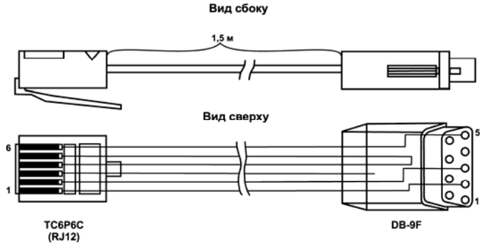
Рисунок Д.1 – Схема кабеля KC1
