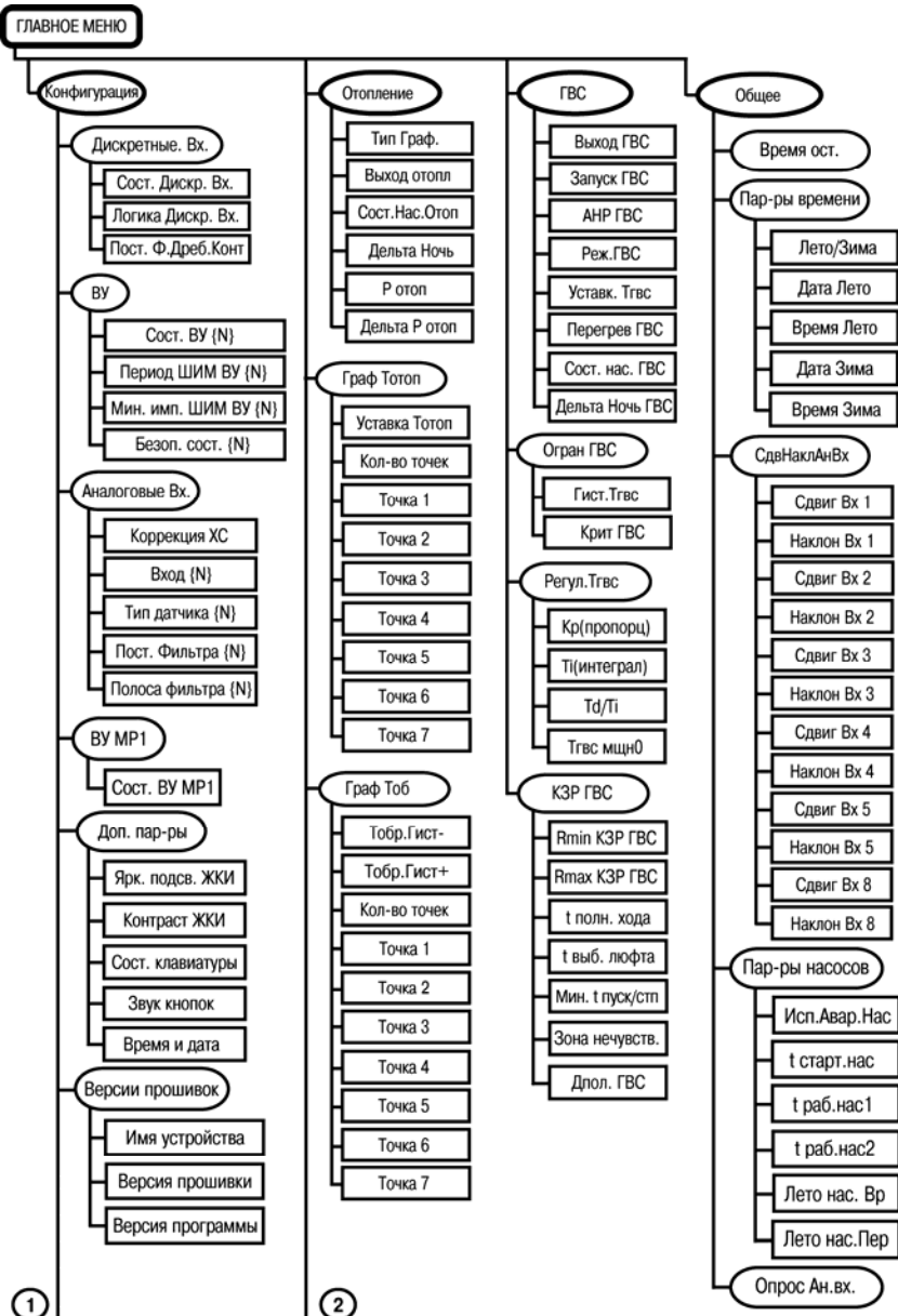
Рисунок И.1 – Главное меню прибора
