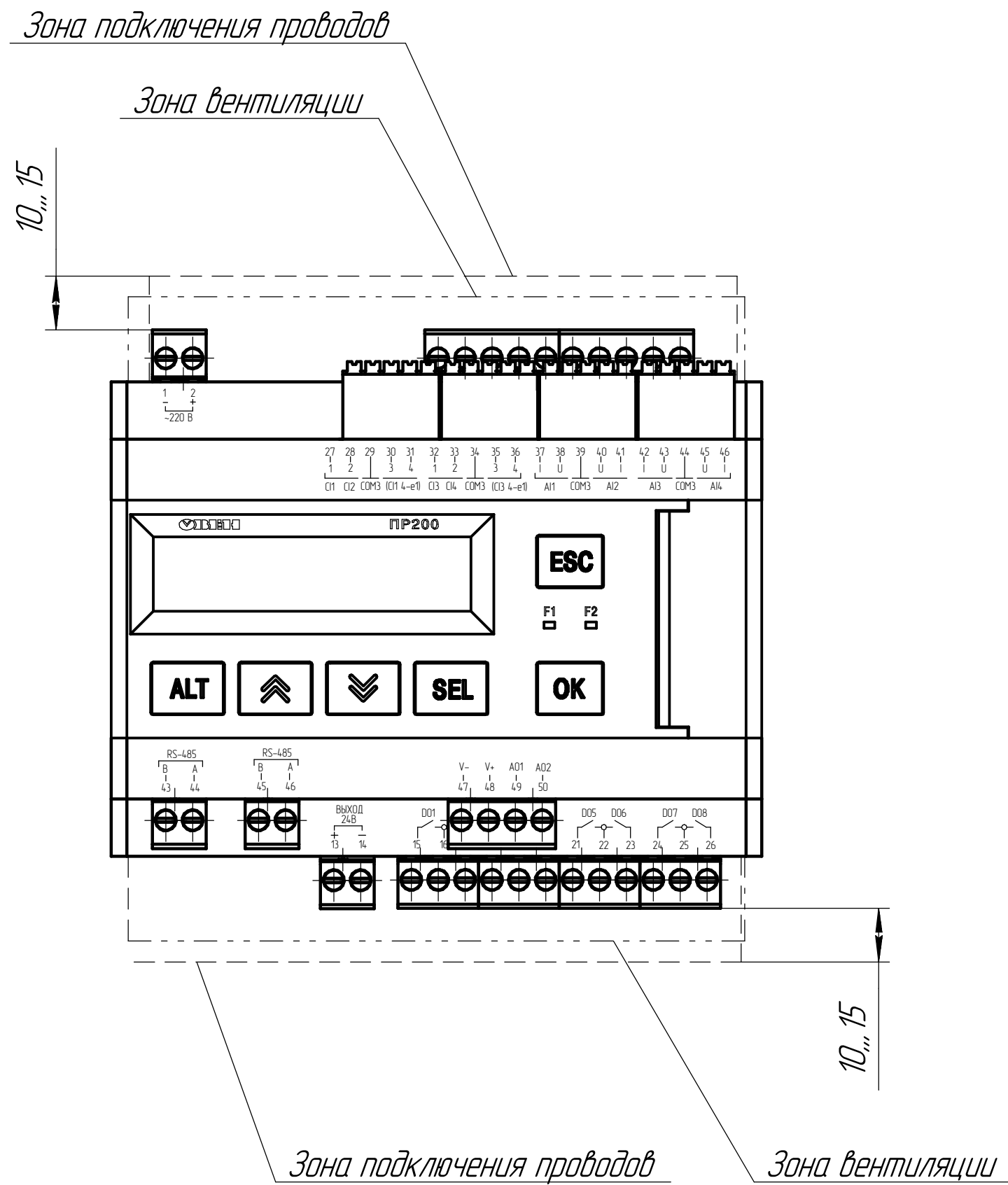
Расположение зон вентиляции и подключения проводов
