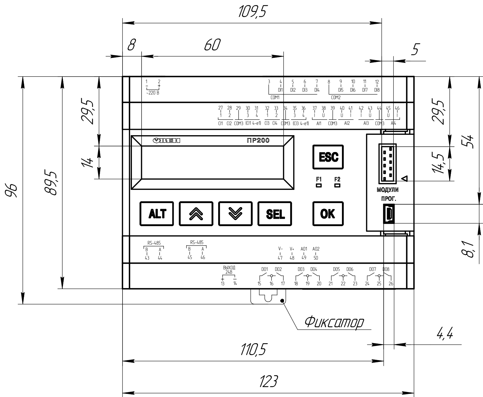
Разъемы клеммные и крышка малая условно не показаны
