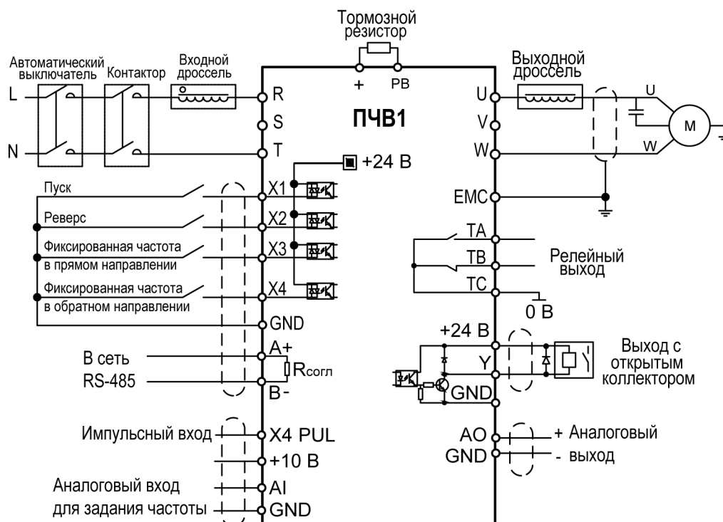
Рисунок 6.6 – Общая схема подключения ПЧВ-X-A [M01] мощностью 0,75 – 2,2 кВт к однофазному конденсаторному электродвигателю
