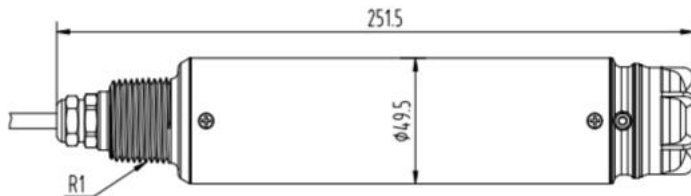
Рисунок 2 – Габаритные размеры
