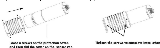
Рисунок 1 – Установка защитного кожуха
