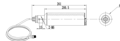
Рисунок 3 – Габаритные размеры датчика в автоматическом очистном устройстве
