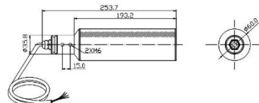
Рисунок 2 – Габаритные размеры датчика без автоматического очистного устройства
