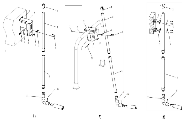
Рисунок 1 – Варианты установки датчика
