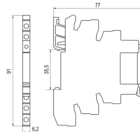
Рисунок 1 – Габаритные размеры
