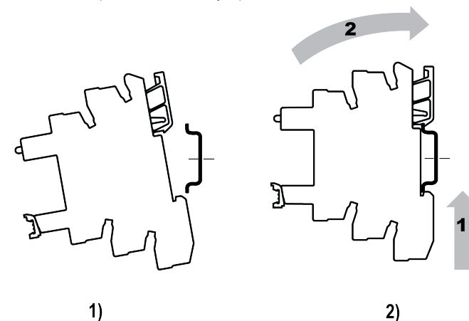
Рисунок 2 – Монтаж
