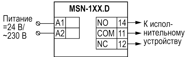
Рисунок 3 – Схема подключения
