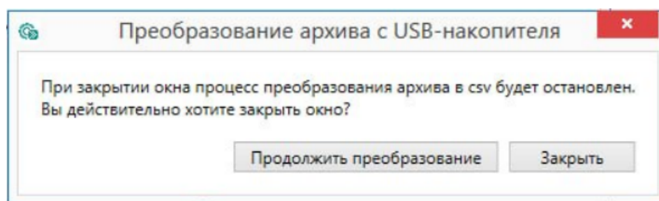
Рисунок 8.27
