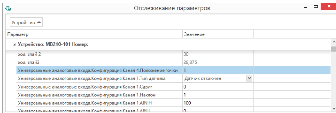
Рисунок 8.4 – Редактирование значения
