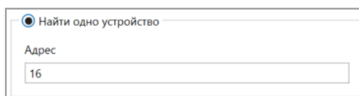
Рисунок 5.27 – Адрес устройства
