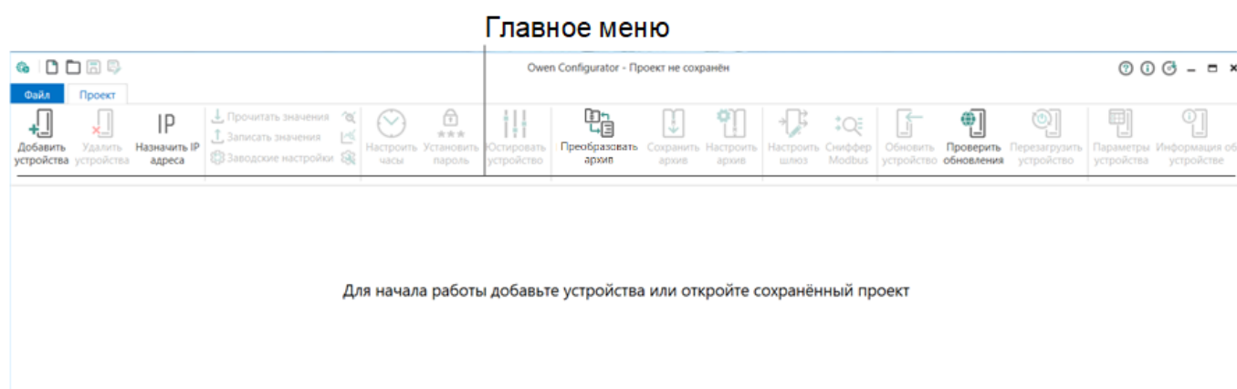
Рисунок 3.1 – Главное окно
