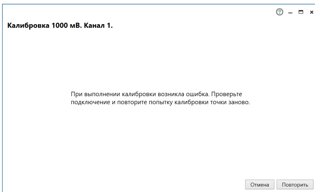
Рисунок 6.14 – Ошибка калибровки
