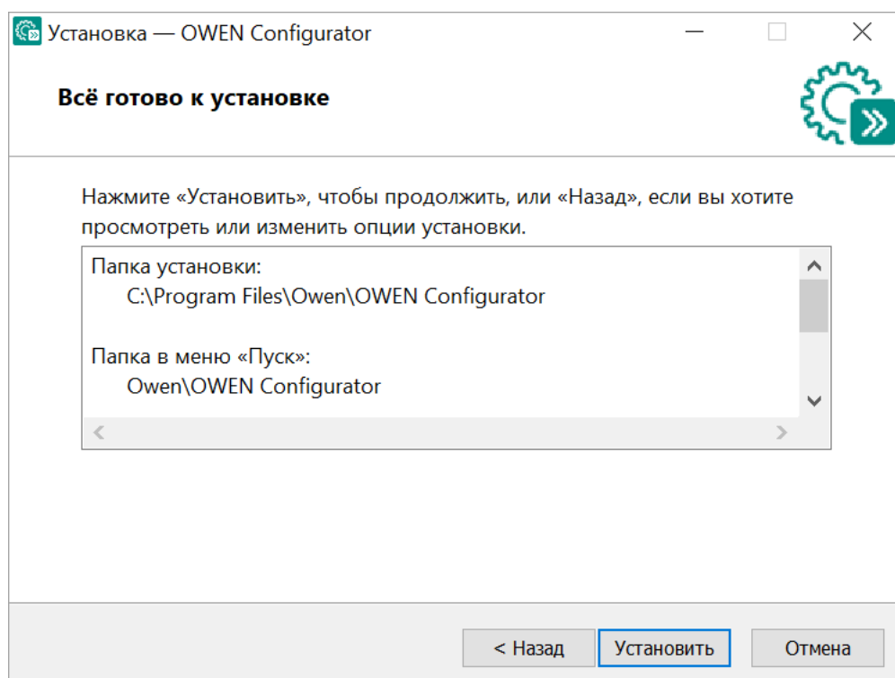
Рисунок 2.7 – Окно установки
