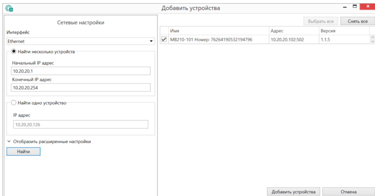
Рисунок 5.5 – Найденные устройства
