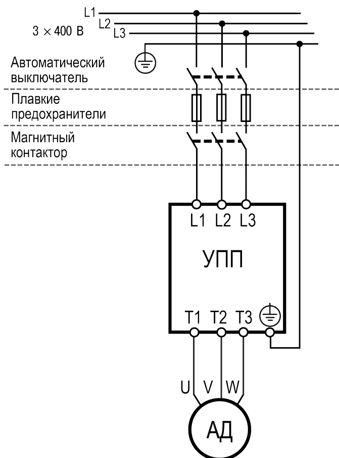
Рисунок 5.1 – Типовая структурная схема электропривода с УПП
