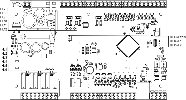
Рисунок 3 – Расположение светодиодов
