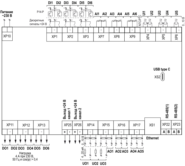
Рисунок 2 – Схема подключения
