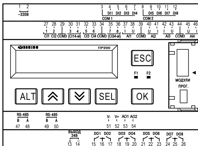
Рисунок А.1 – Расположение контактов ПР200-220.28.2.X
