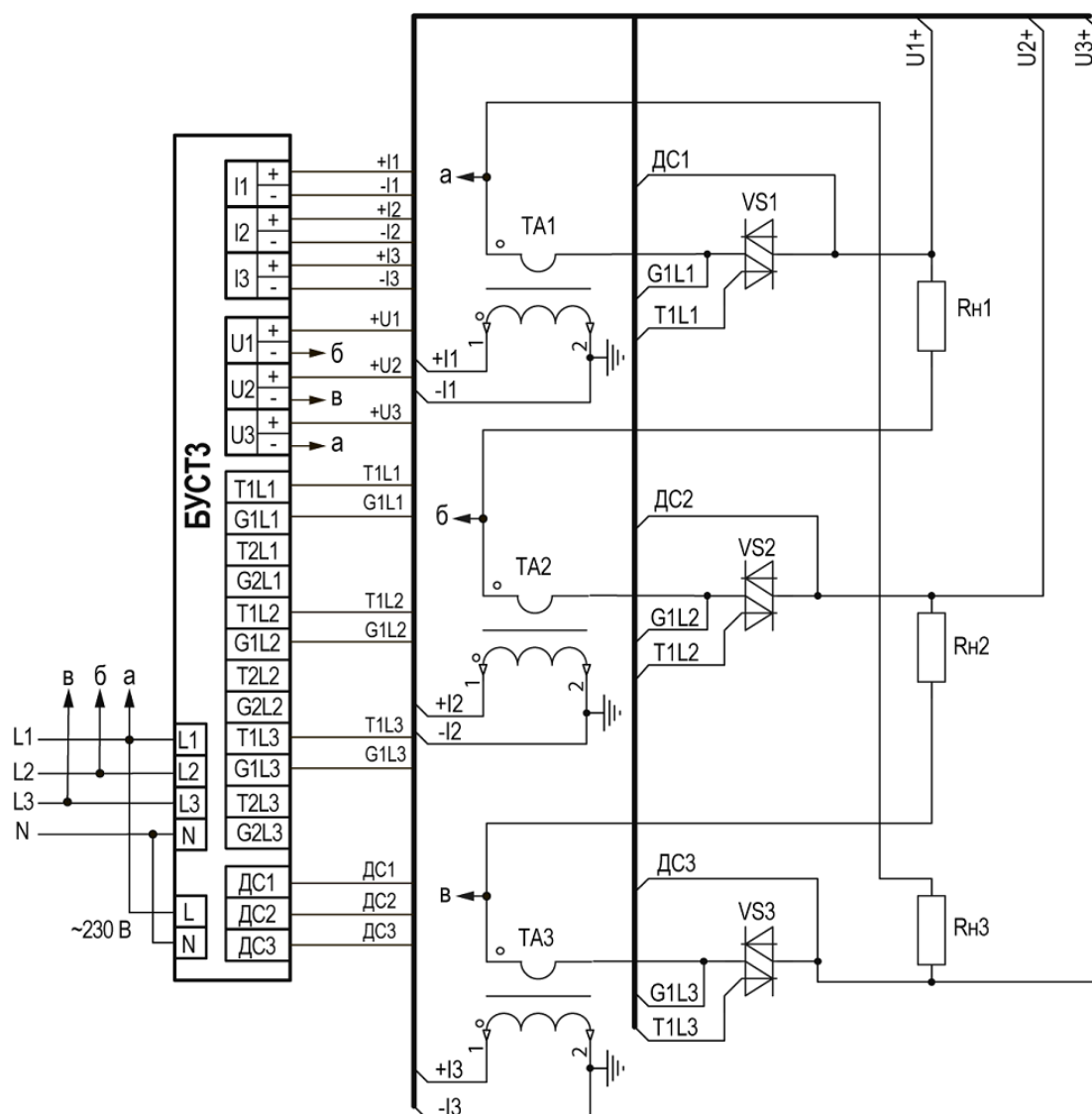
Рисунок 5.8 – Схема подключения симисторов по схеме «разомкнутый треугольник»
