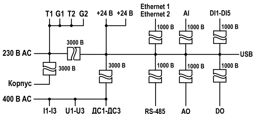
Рисунок 2.1 – Схема гальванической развязки
