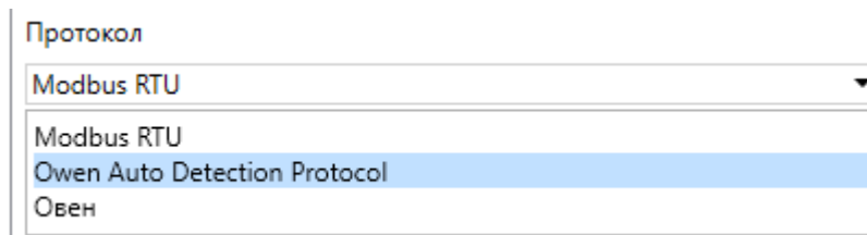
Рисунок 7.4 – Выбор протокола
