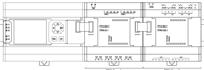
Рисунок 14 – Расположение модулей расширения на шине
