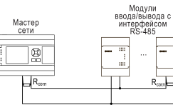
Рисунок 13 – Типовая схема подключения в режиме Master
