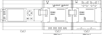
Рисунок 13 – Расположение модулей расширения на шине
