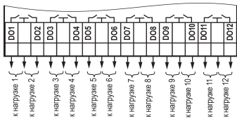
Рисунок 9 – Схема подключения ВЭ типа «Р»
