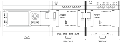
Рисунок 13 – Расположение модулей расширения на шине
