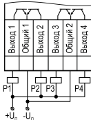
Рисунок 9 – Схема подключения нагрузок типа «КТ»
