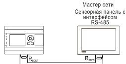
Рисунок 11 – Типовая схема подключения в режиме Slave
