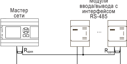
Рисунок 12 – Типовая схема подключения в режиме Master
