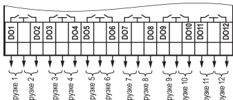
Рисунок 8 – Схема подключения ВЭ типа «Р»
