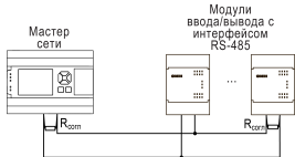
Рисунок 13 – Типовая схема подключения в режиме Master
