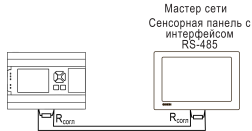
Рисунок 12 – Типовая схема подключения в режиме Slave
