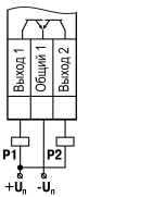
Рисунок 8 – Схема подключения нагрузок типа «КТ»
