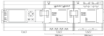
Рисунок 15 – Расположение модулей расширения на шине
