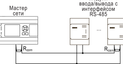
Рисунок 13 – Типовая схема подключения в режиме Master
