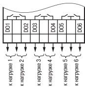
Рисунок 9 – Схема подключения ВЗ типа «Р»
