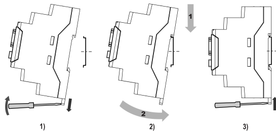
Рисунок 2 – Монтаж прибора
