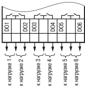
Рисунок 9 – Схема подключения ВЭ типа «Р»
