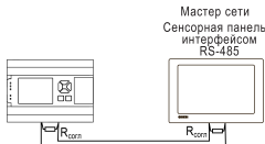
Рисунок 11 – Типовая схема подключения в режиме Slave
