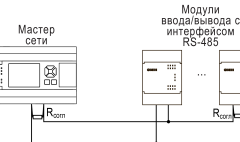
Рисунок 12 – Типовая схема подключения в режиме Master
