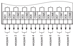
Рисунок 8 – Схема подключения нагрузок к ВЗ типа «Р»
