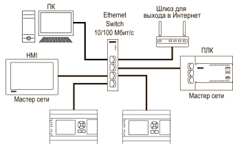
Рисунок 13 – Подключение по схеме «Звезда»
