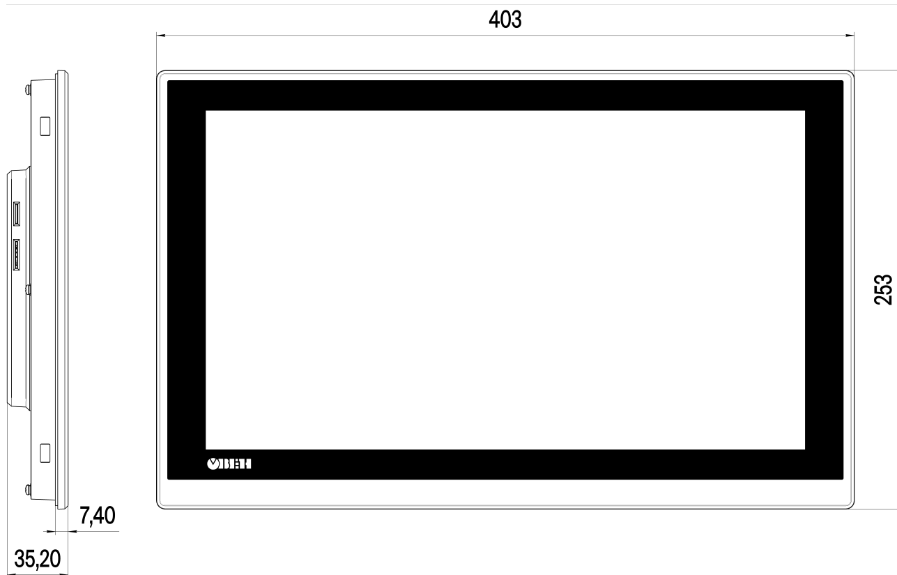
Рисунок 4.8 – Габаритные размеры СПК210-15
