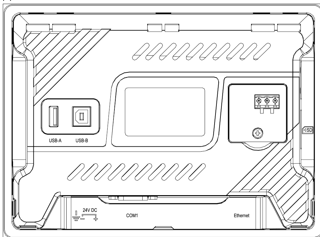
Рисунок 5.1 – Внешний вид задней стороны СПК210-07
