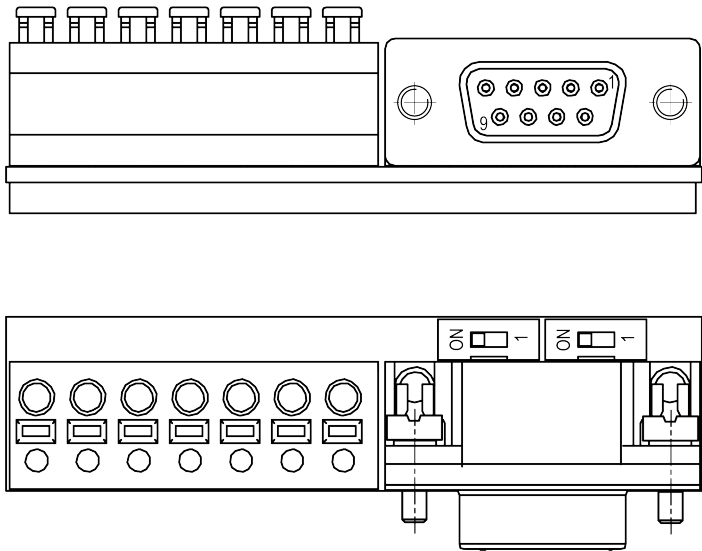
Рисунок 5.5 – Внешний вид адаптера СПК210 для модификаций СПК210–07 и СПК210–10
