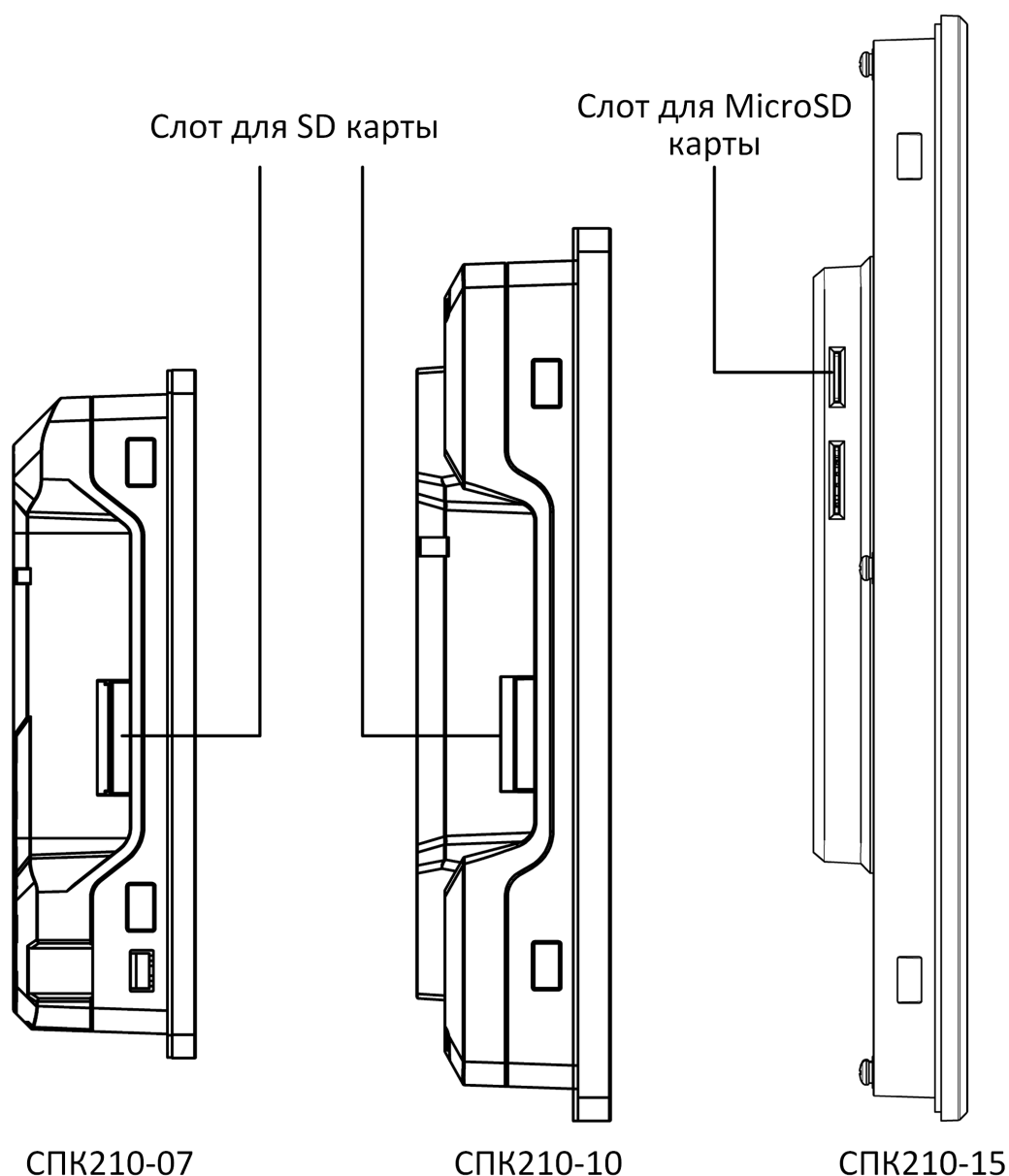
Рисунок 5.11 – Внешний вид боковой грани
