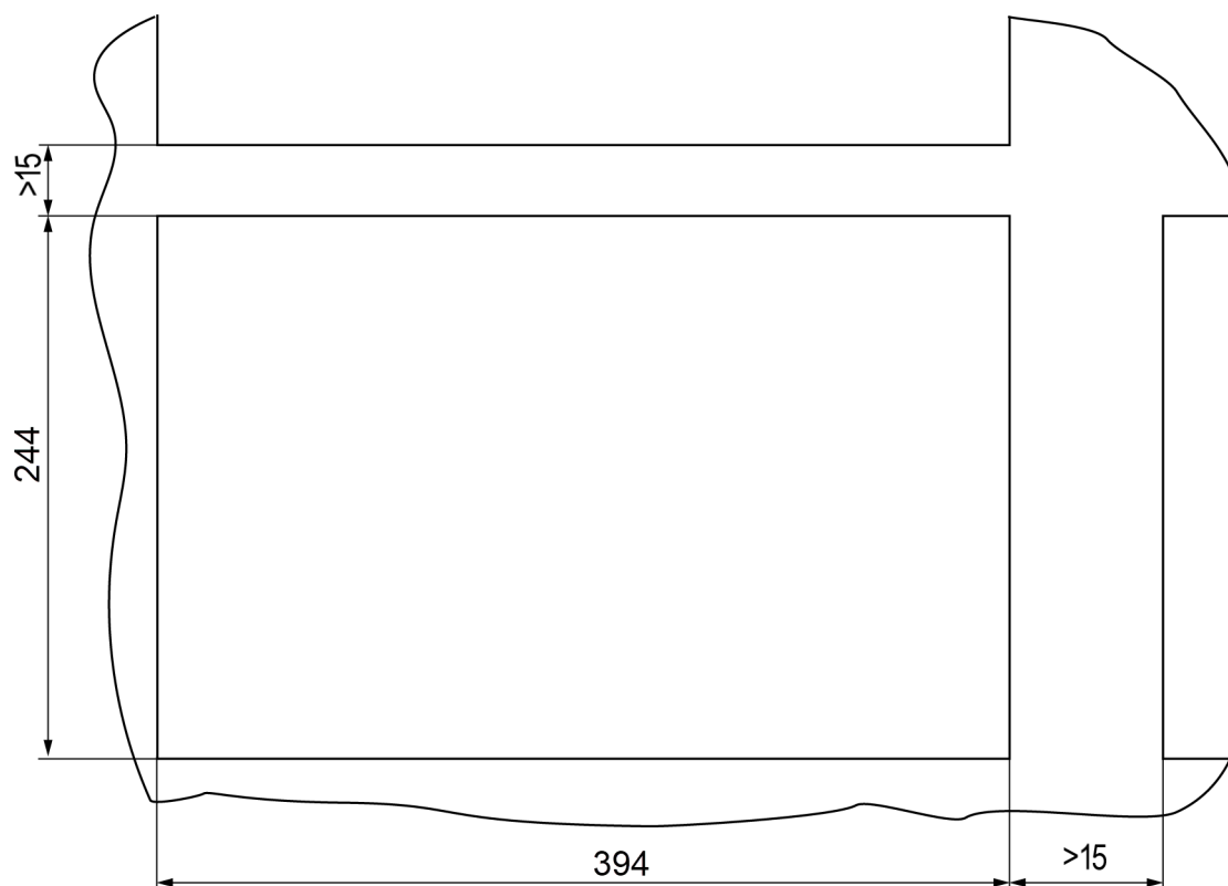
Рисунок 4.9 – Установочные размеры СПК210-15
