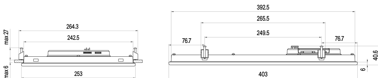
Рисунок 4.10 – Дополнительные установочные размеры СПК210-15
