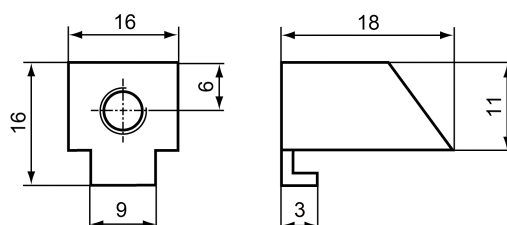
Рисунок 4.7 – Размеры крепежа
