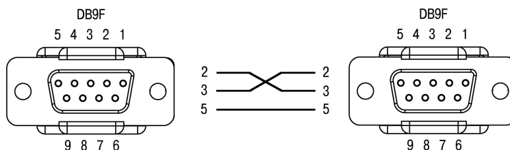
Рисунок 5.4 – Схема нуль-модемного кабеля для подключения по порту RS-232
