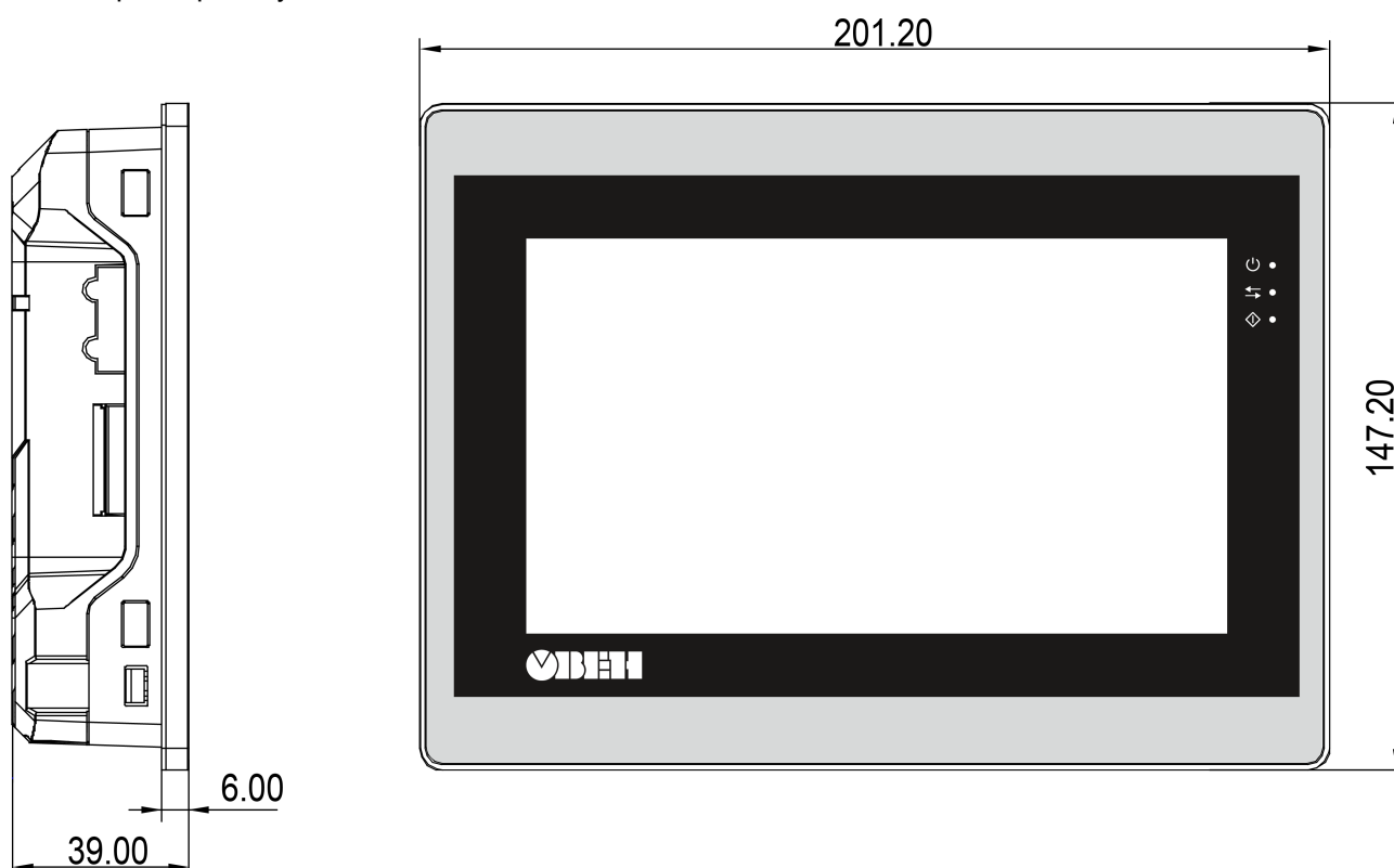
Рисунок 4.1 – Габаритные размеры СПК210-07
