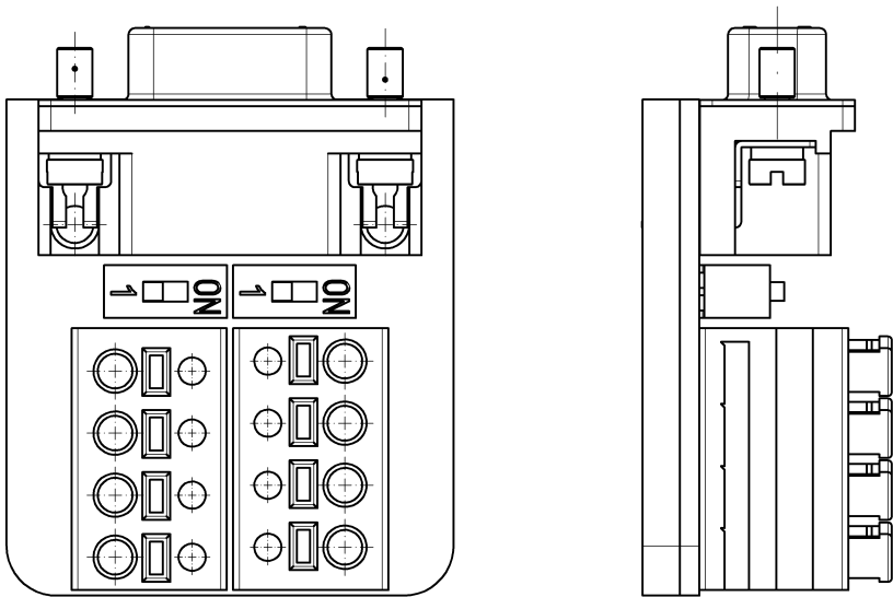
Рисунок 5.6 – Внешний вид адаптера СПК210 для модификации СПК210–15
