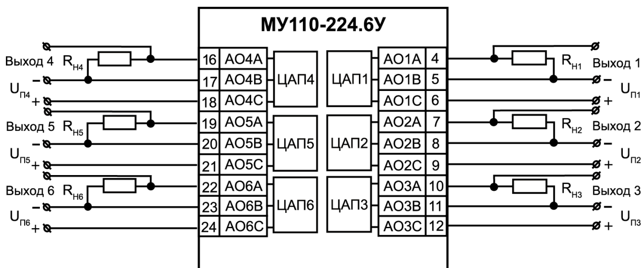
Рисунок 5.3 – Схема подключения нагрузки к аналоговым выходам
