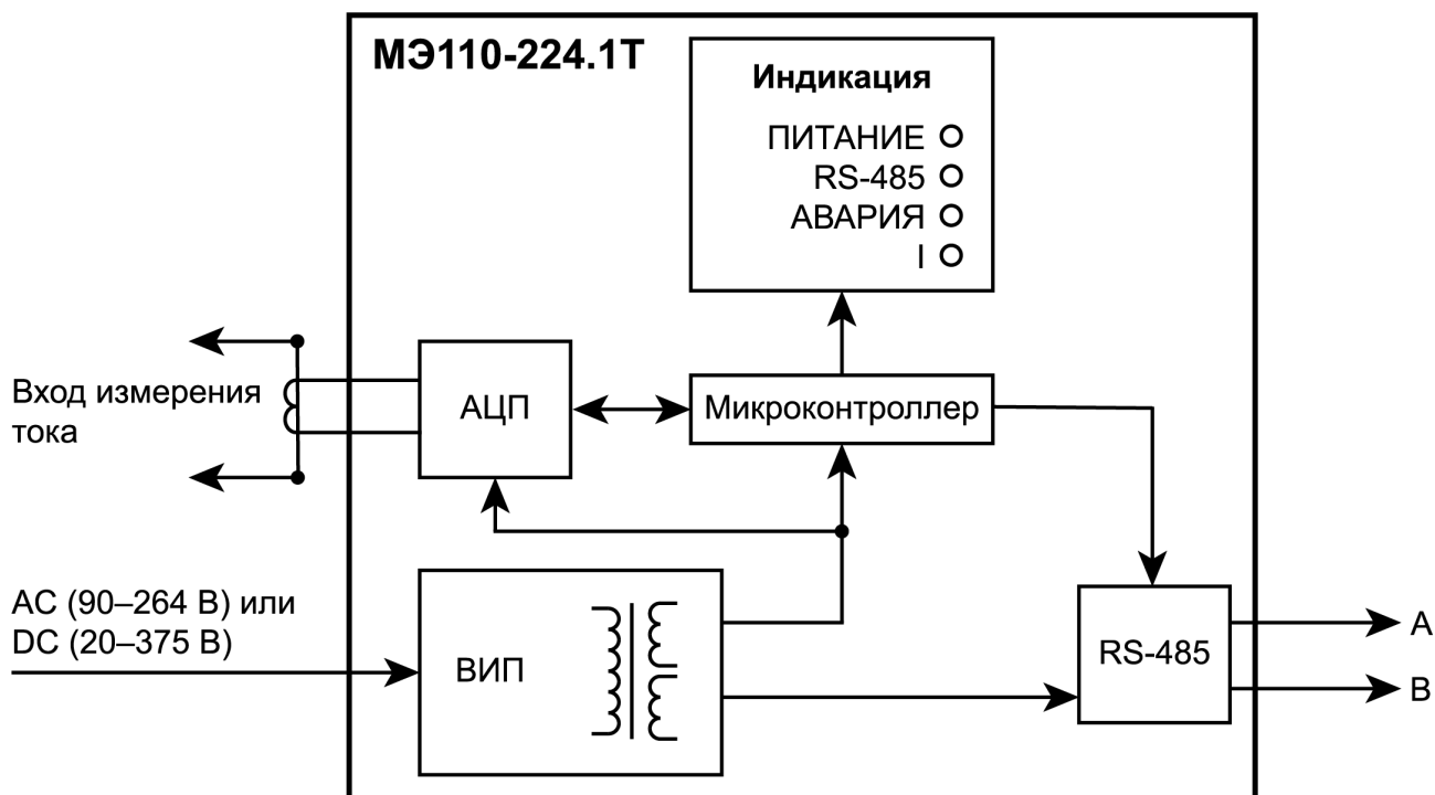
Рисунок 6.1 – Структурная схема прибора
