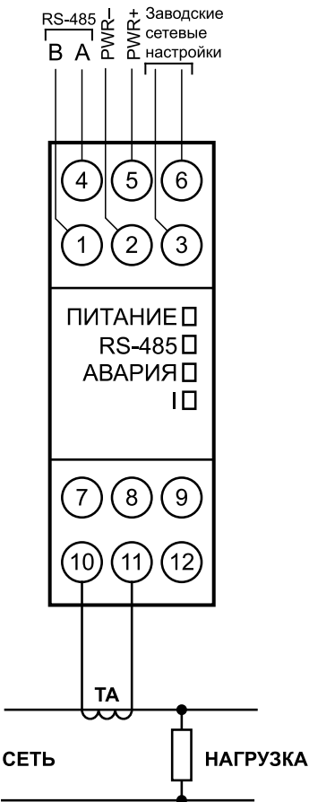
Рисунок 5.2 – Подключение прибора к однофазной сети через согласующий трансформатор
