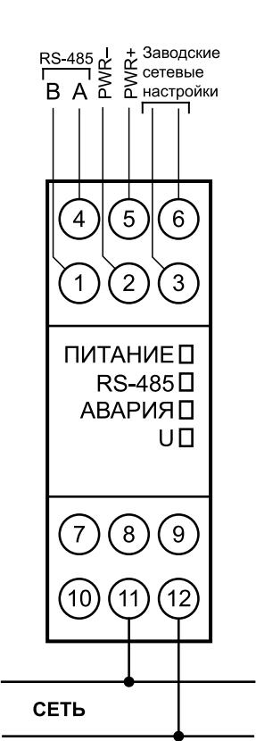
Рисунок 5.1 – Подключение прибора к однофазной сети
