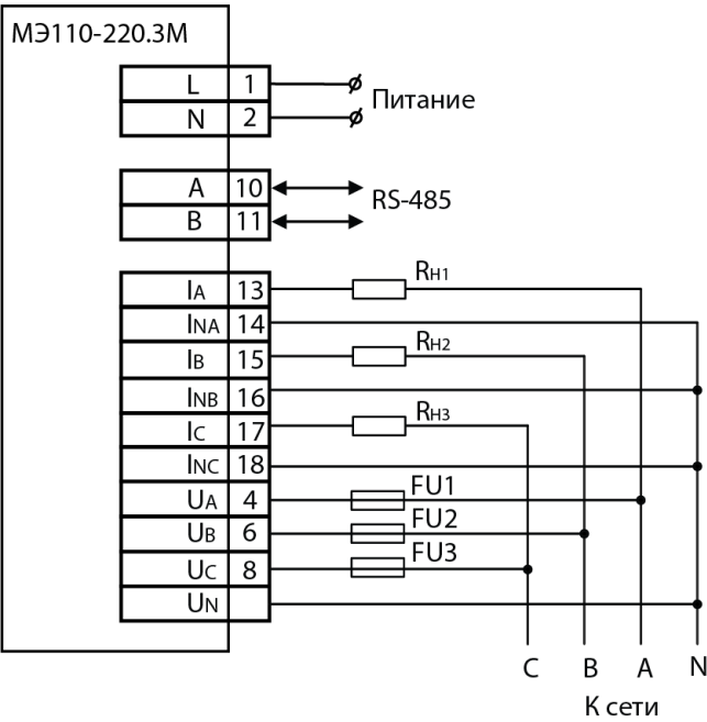
Рисунок 5.3 – Подключение прибора к трехфазной сети
