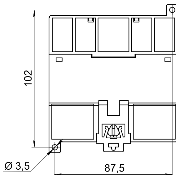
Рисунок 4.2 – Установочные размеры
