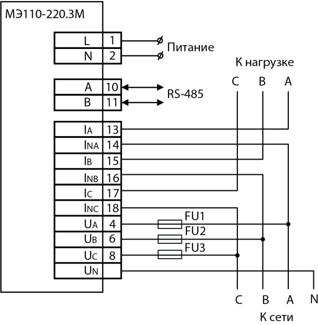
Рисунок 5.4 – Подключение к прибору нагрузки без нейтрали
