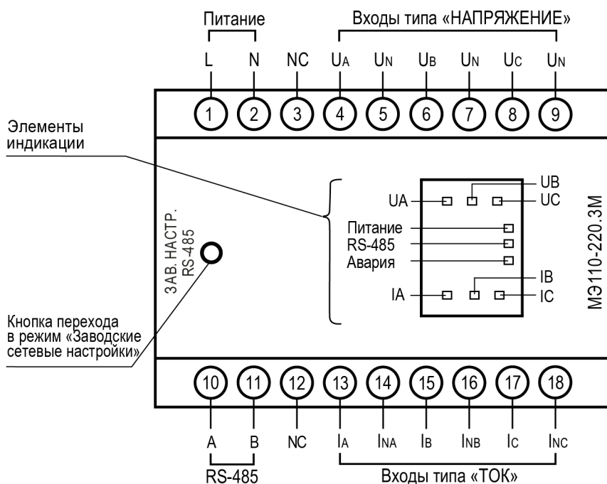
Рисунок 5.2 – Общий вид
