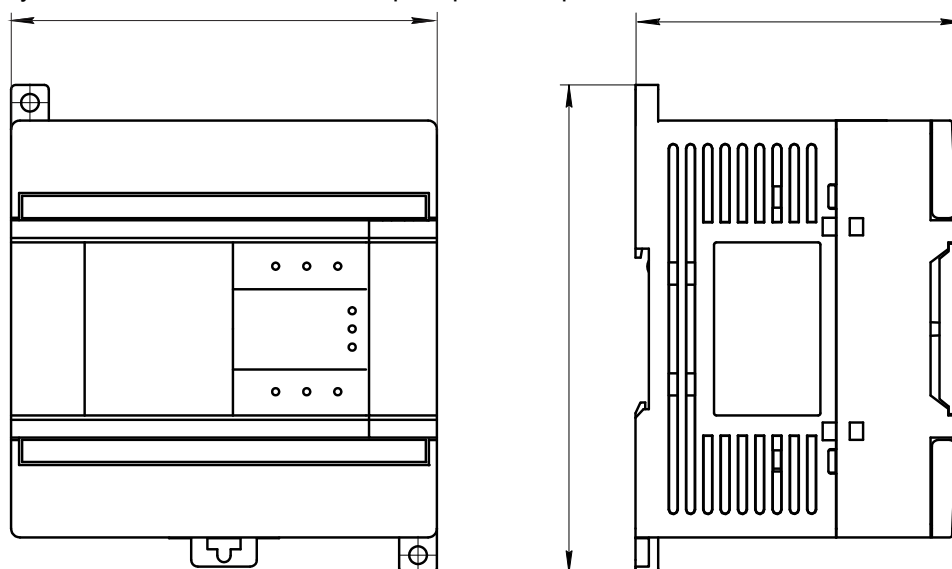
Рисунок 4.1 – Габаритные размеры
