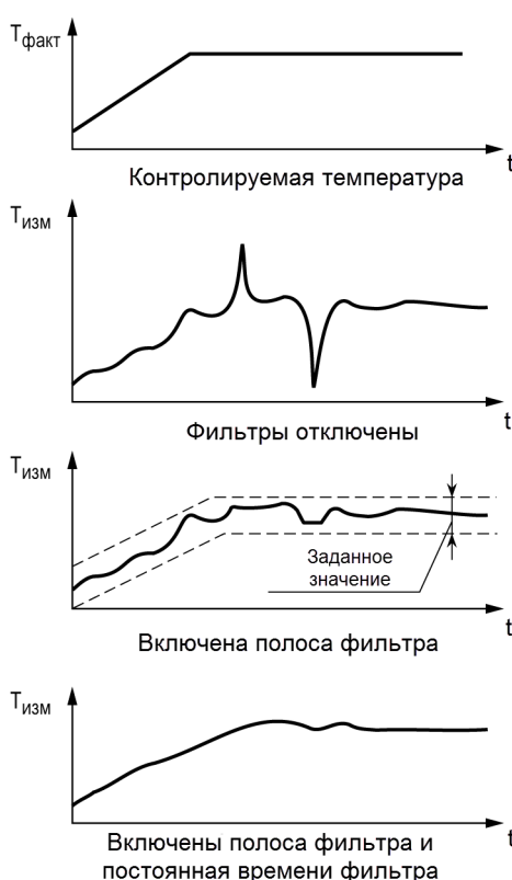
Рисунок 5.26 – Временные диаграммы работы цифровых фильтров
