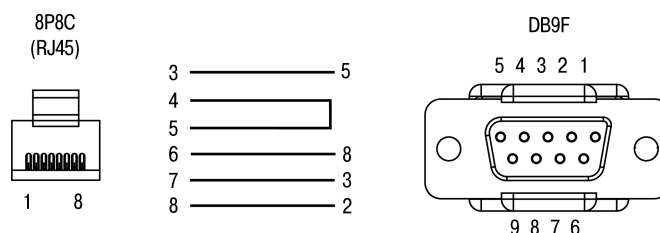
Рисунок 5.30 – Схема кабеля KC14
