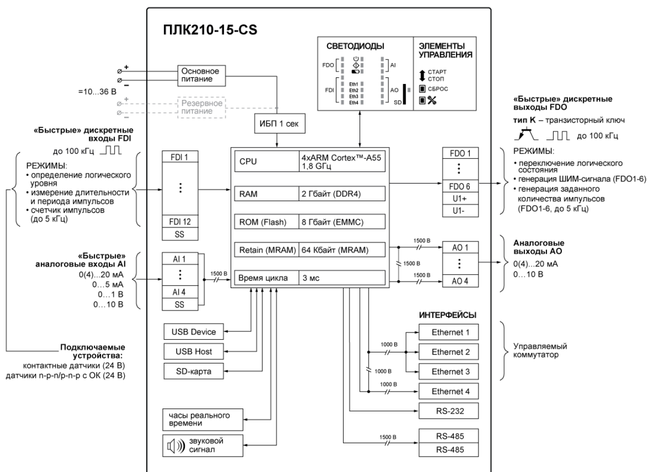
Рисунок 3.5 – Функциональная схема ПЛК210-15-CS
