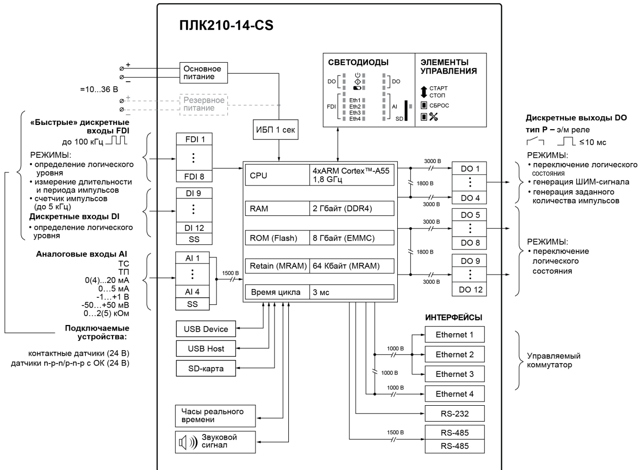
Рисунок 3.4 – Функциональная схема ПЛК210-14-CS
