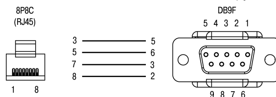
Рисунок 5.31 – Схема кабеля KC16
