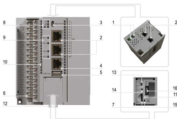
Рисунок 3.7 – Внешний вид ПЛК210 (модификации 11, 12, 13, 14, 15)
