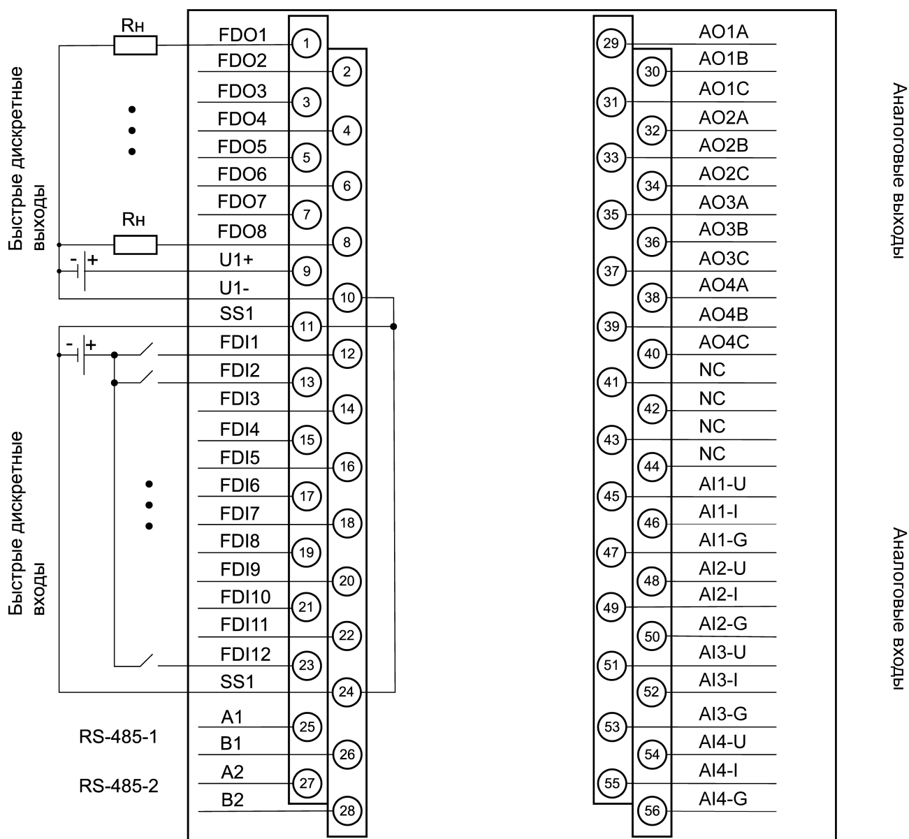
Рисунок 5.6 – Назначение контактов клеммника (модификация 15)
