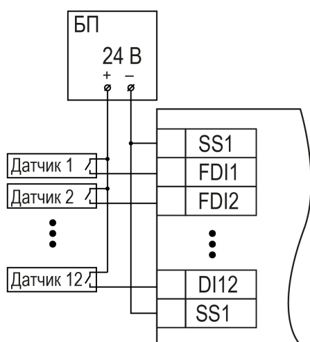
Рисунок 5.8 – Схема подключения контактных датчиков к дискретным входам FDI1–FDI8, DI9–DI12
