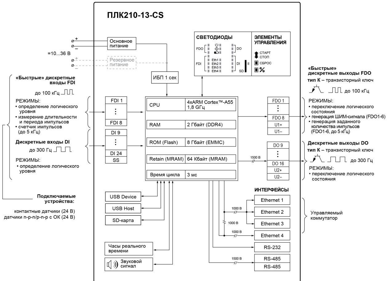
Рисунок 3.3 – Функциональная схема ПЛК210-13-CS
