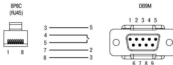
Рисунок 5.32 – Схема кабеля KC17
