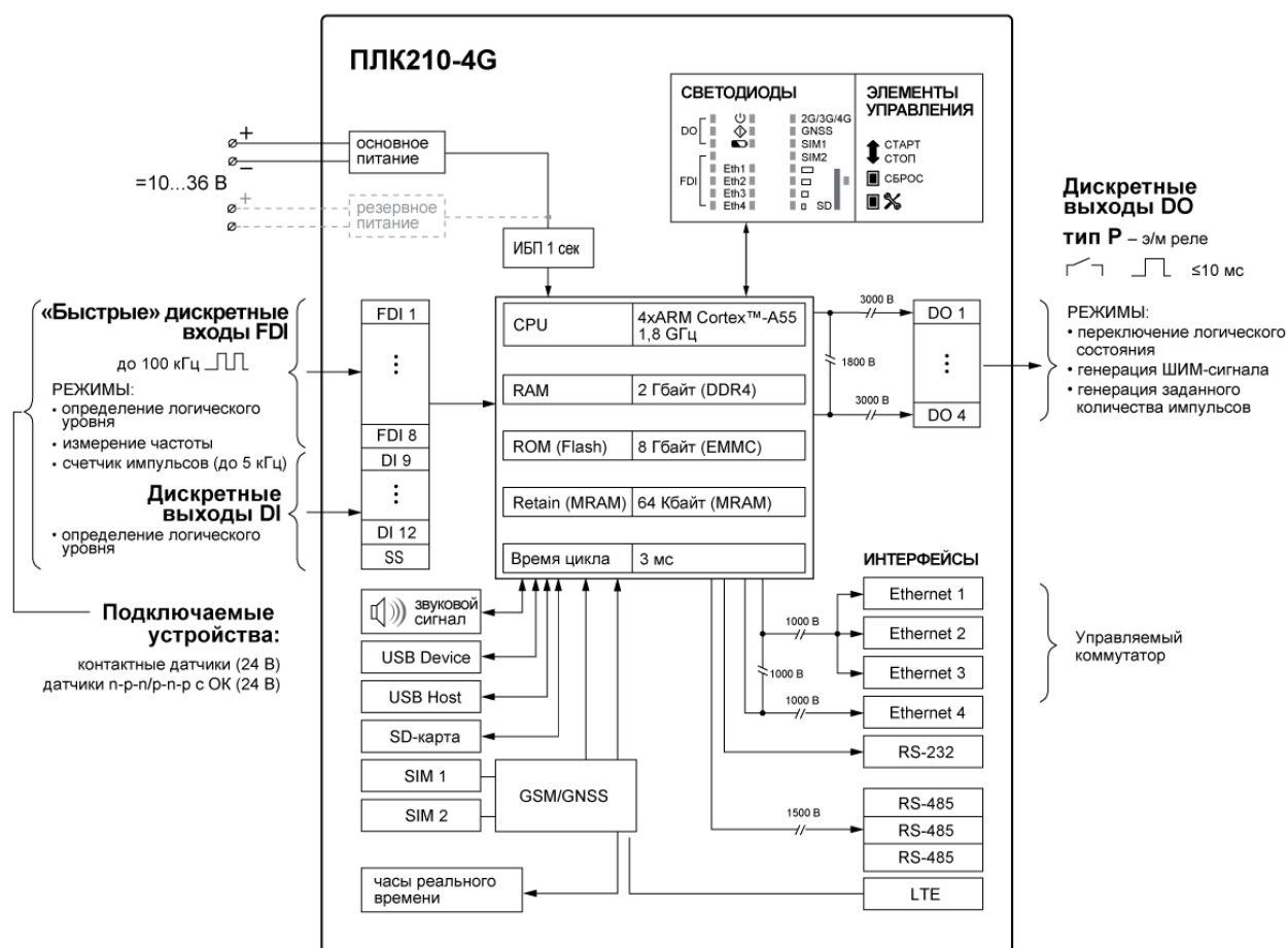
Рисунок 3.6 – Функциональная схема ПЛК210-4G-CS
