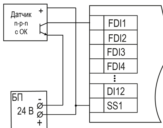
Рисунок 5.11 – Подключение транзисторов типа п-р-п* к дискретным входам FDI1–FDI8, DI9–DI12
