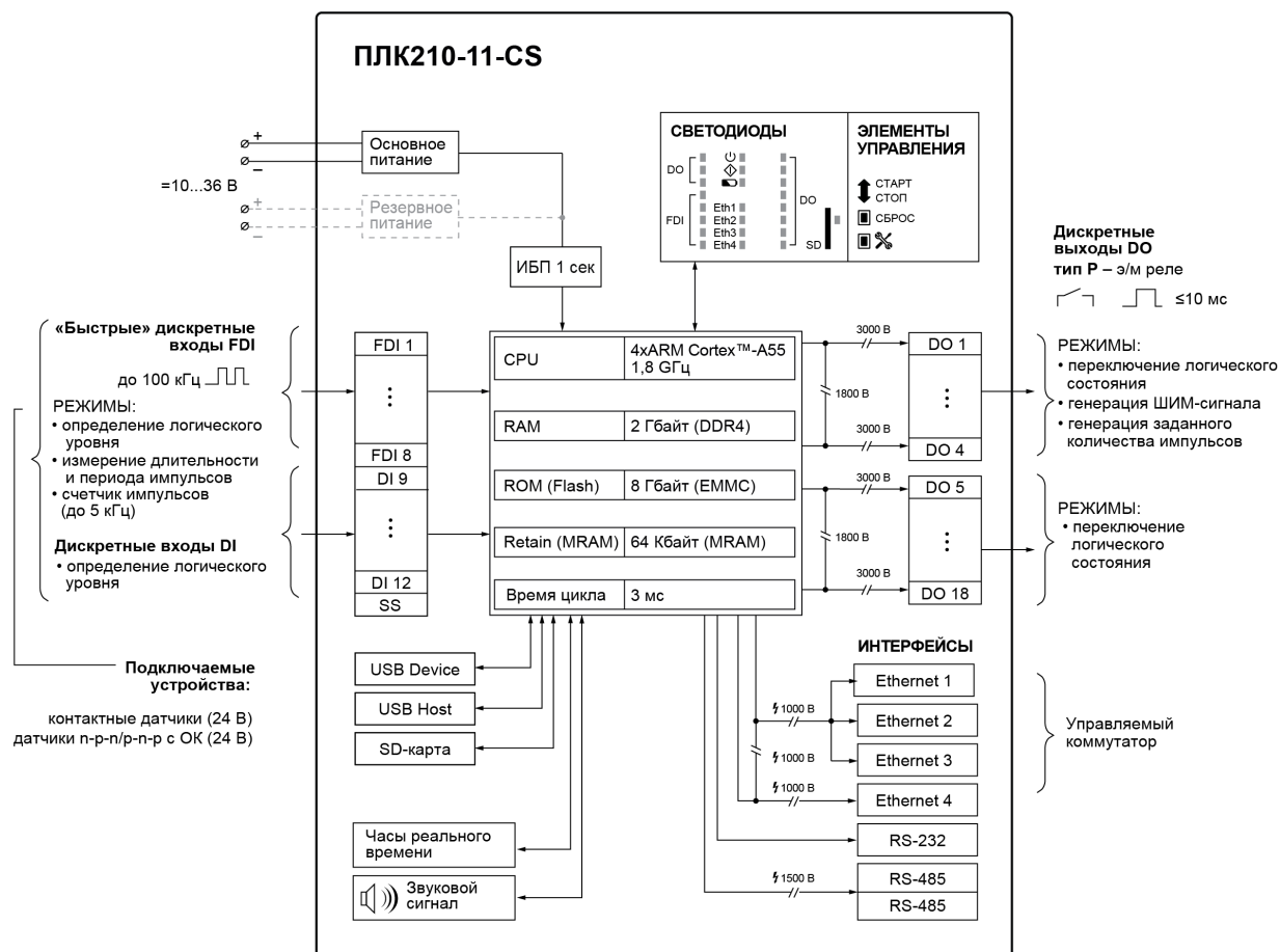
Рисунок 3.1 – Функциональная схема ПЛК210-11-CS
