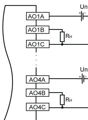
Рисунок 5.17 – Схема подключения нагрузки к аналоговым выходам
