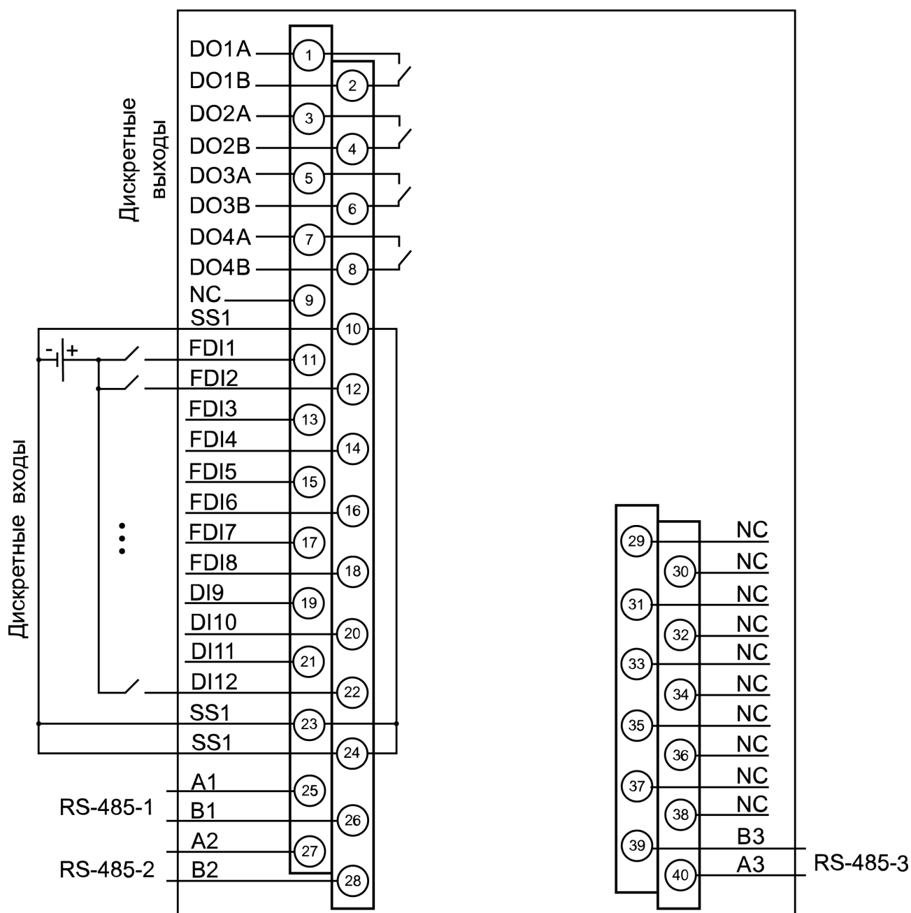
Рисунок 5.7 – Назначение контактов клеммника (модификация 4G)
