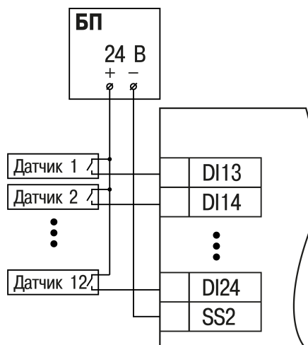
Рисунок 5.9 – Схема подключения контактных датчиков к дискретным входам DI13–DI24 (модификация 12)
