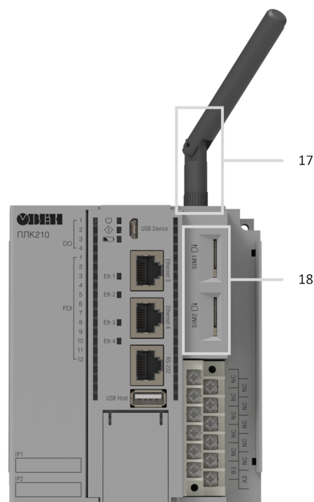
Рисунок 3.8 – Внешний вид ПЛК210-4G
