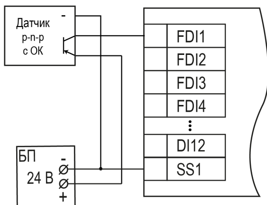
Рисунок 5.10 – Подключение транзисторов типа р-п-р к дискретным входам FDI1–FDI8, DI9–DI12
