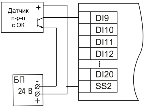
Рисунок 5.11 – Подключение транзисторов типа n-р-n DI9–DI20
