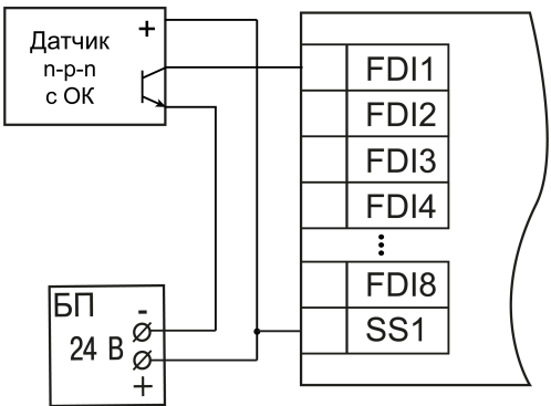
Рисунок 5.9 – Подключение транзисторов типа n-р-n* FDI1–FDI8
