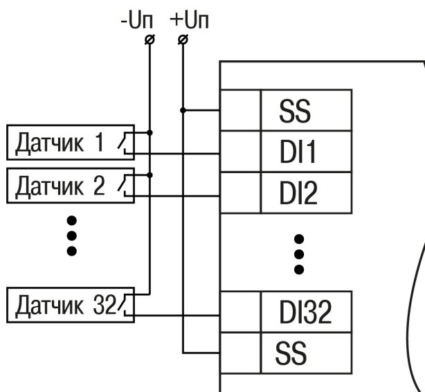
Рисунок 5.4 – Схема подключения к входам DI1–DI32 – вариант 1 (MB210-212)
