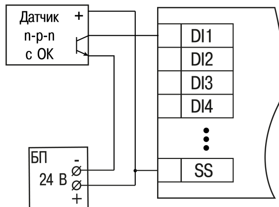
Рисунок 5.8 – Подключение транзисторов п-р-п (MB210-212)
