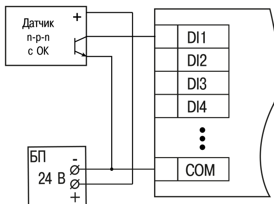
Рисунок 5.9 – Подключение транзисторов п-р-п (MB210-204)
