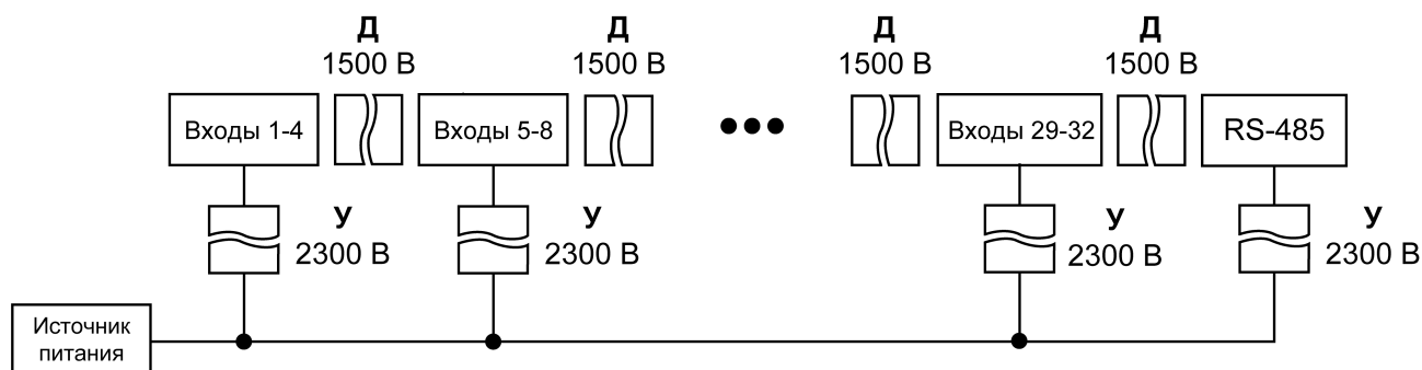
Рисунок 2.1 – Изоляция узлов модуля MB110-32ДН
