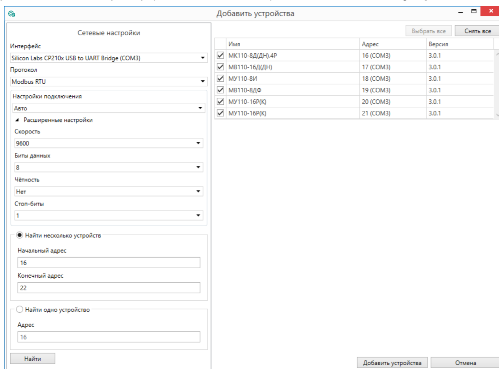
Рисунок 8.1 – Настройка сетевых параметров в ПО OWEN Configurator
