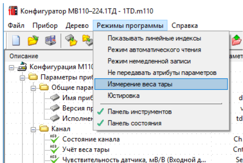
Рисунок 8.4 – Автоматическое измерение веса тары
