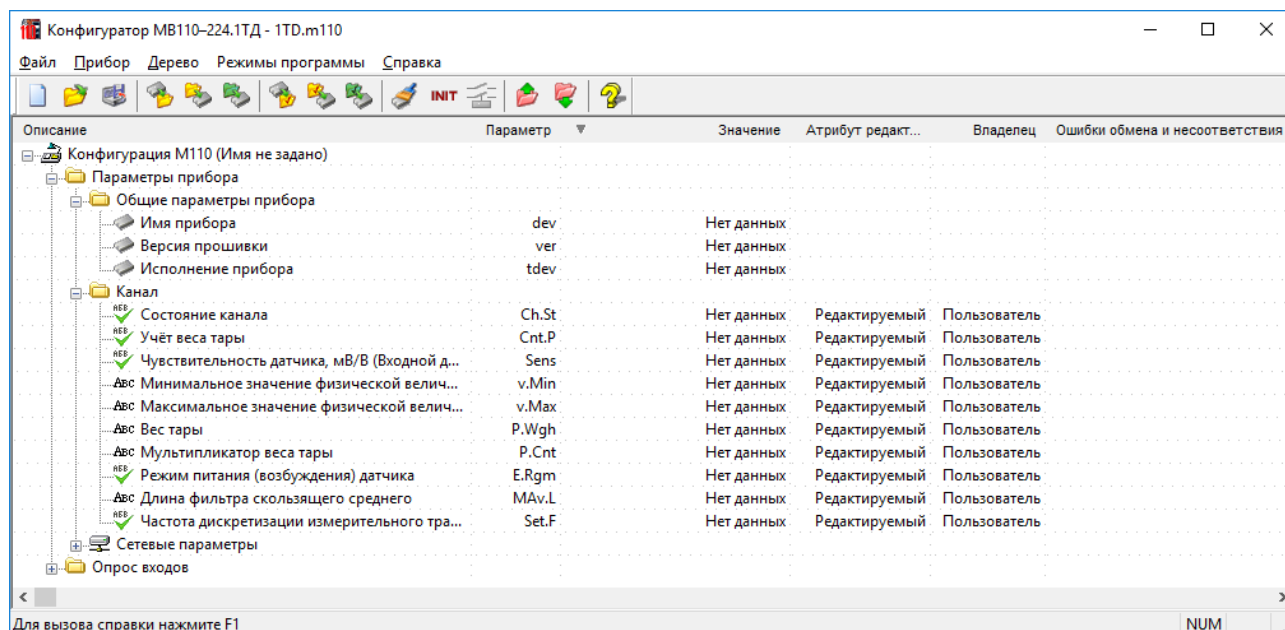
Рисунок 8.2 – Конфигурационные параметры прибора
