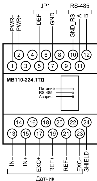
Рисунок 5.2 – Назначение контактов клеммной колодки MB110-224.1ТД
