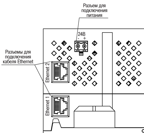
Рисунок 5.2 – Разъемы прибора
