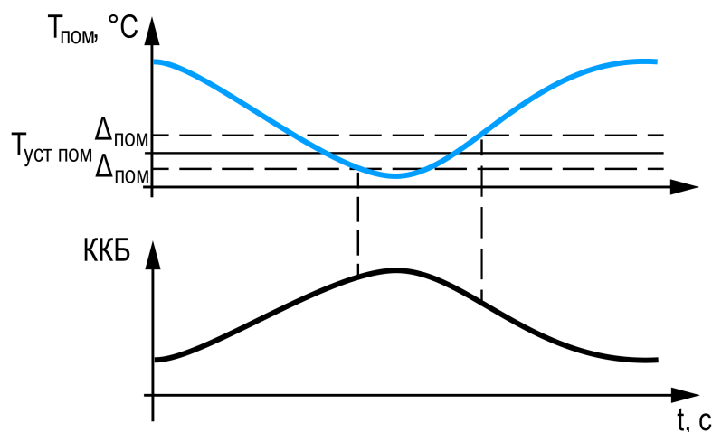
Рисунок 10.18 – Плавное управление ККБ
