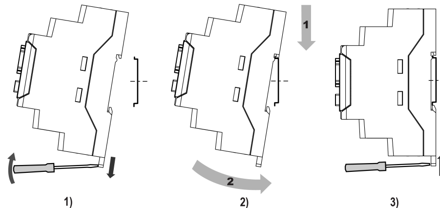
Рисунок 5.2 – Монтаж прибора
