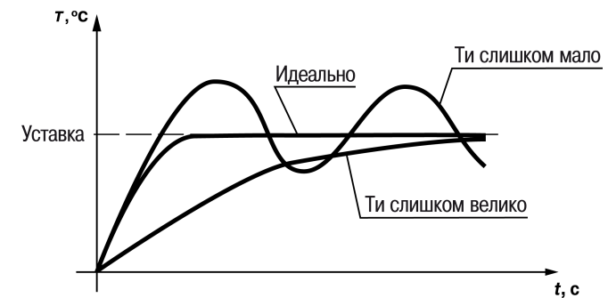
Рисунок 10.22 – Влияние T и на выход на уставку
