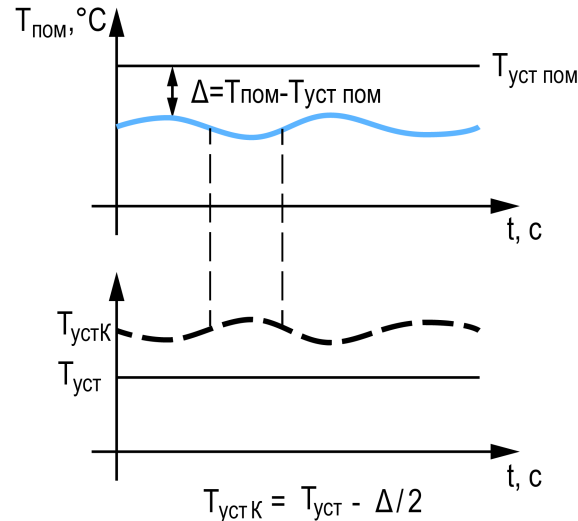
Рисунок 10.20 – Каскадное регулирование
