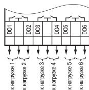
Рисунок 10 – Схема подключения ВЭ типа «Р»
