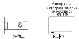
Рисунок 12 – Типовая схема подключения в режиме Slave
