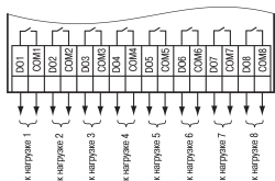
Рисунок 8 – Схема подключения нагрузок к ВЭ типа «P»
