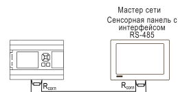
Рисунок 11 – Типовая схема подключения в режиме Slave
