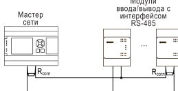
Рисунок 12 – Типовая схема подключения в режиме Master
