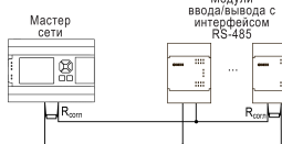
Рисунок 13 – Типовая схема подключения в режиме Master
