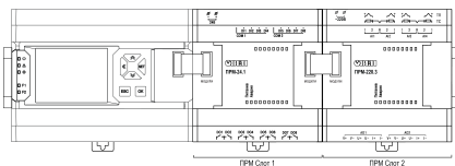
Рисунок 15 – Расположение модулей расширения на шине
