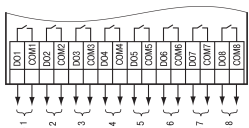
Рисунок 8 – Схема подключения нагрузок к ВЭ типа «Р»
