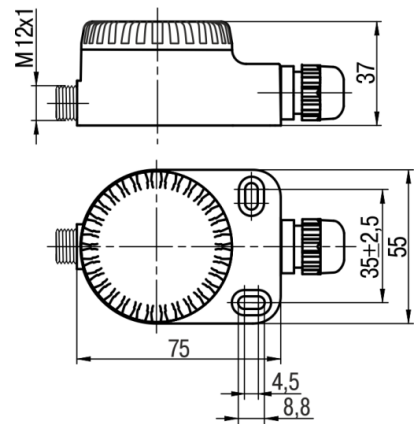
Рисунок Г.6 – Увеличенная пластмассовая коммутационная головка
