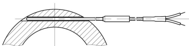
Рисунок 5.9 – Способ монтажа датчика на основе КТМС в паз в цилиндрической поверхности
