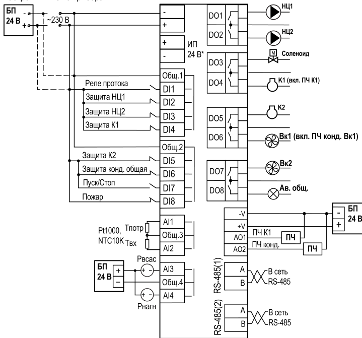
Рисунок 3 – Схема подключения сигналов (пример)
