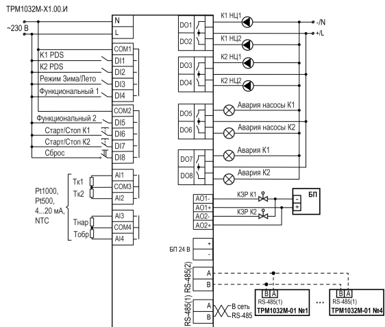
Рисунок 2 – Схема подключения
