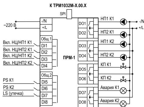
Рисунок 2 – Схема подключения
