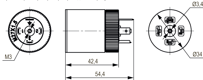
Рисунок 1 – Габаритные размеры прибора
