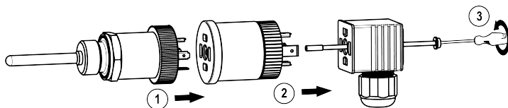
Рисунок 3 – Монтаж прибора
