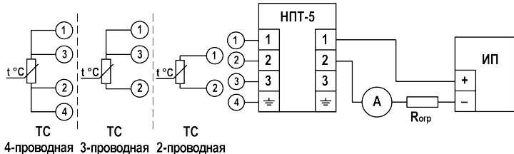
Рисунок 4 – Подключения прибора
