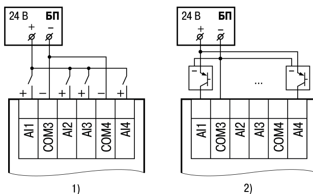
Рисунок 6.8 – Схема подключения к аналоговым входам, работающим в дискретном режиме: 1) датчиков типа «сухой» контакт, 2) трехпроводных дискретных датчиков, имеющих выходной транзистор р-п-типа с открытым коллектором
