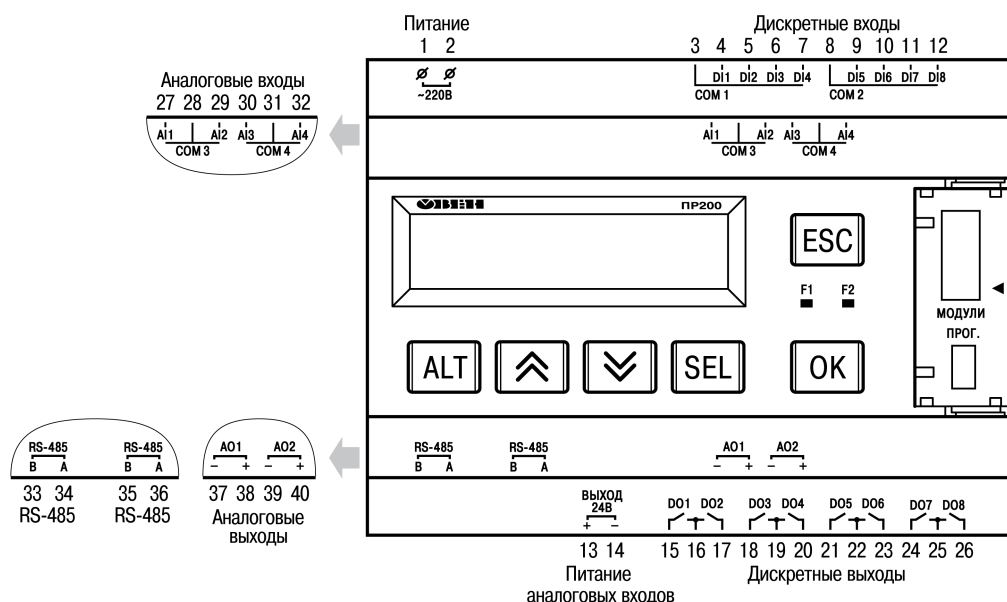
Рисунок А.4 – Расположение контактов ПР200-220.2.2.X
