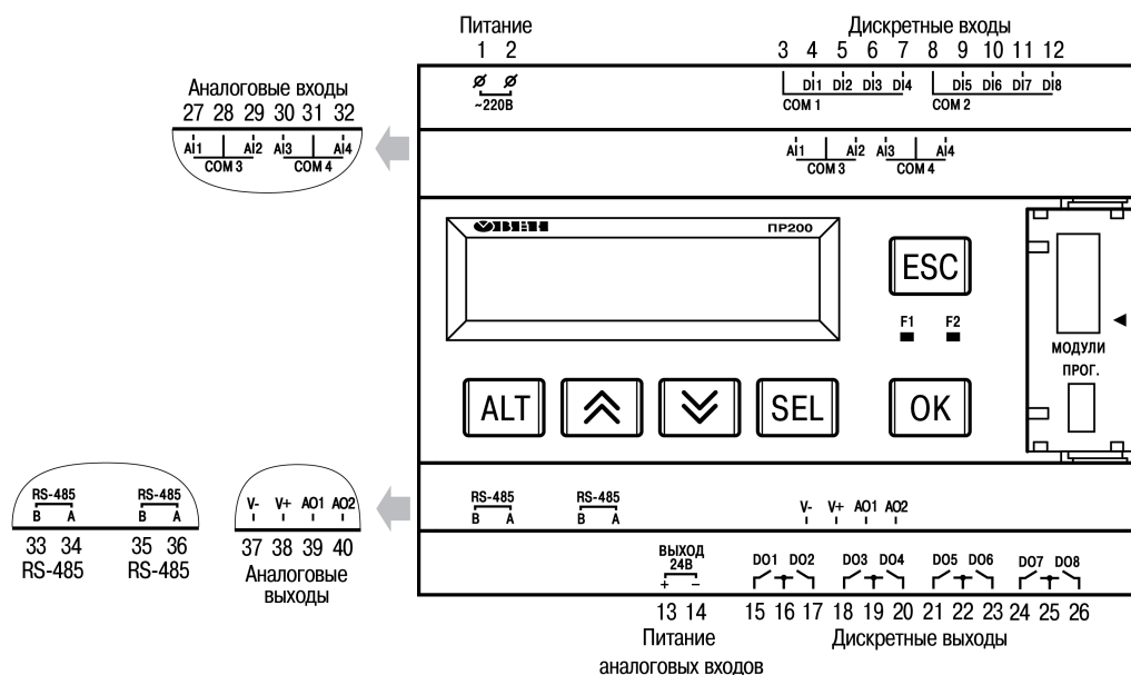
Рисунок А.7 – Расположение контактов PR200-220.4.2.X
