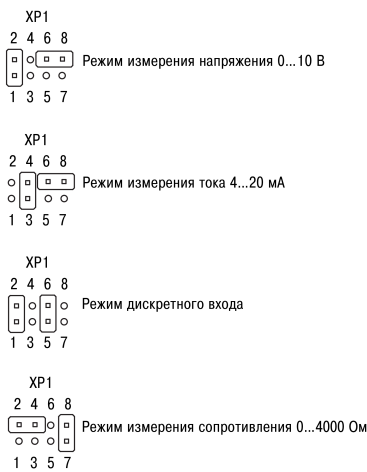
Рисунок 4 – Схема настройки AI1...AI4
