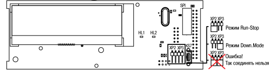
Рисунок 5 – Вид на верхнюю плату со снятой крышкой
