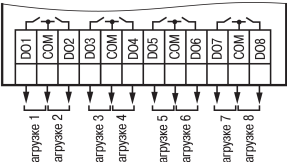
Рисунок 8 – Подключение нагрузки к ВЭ типа «Р»
